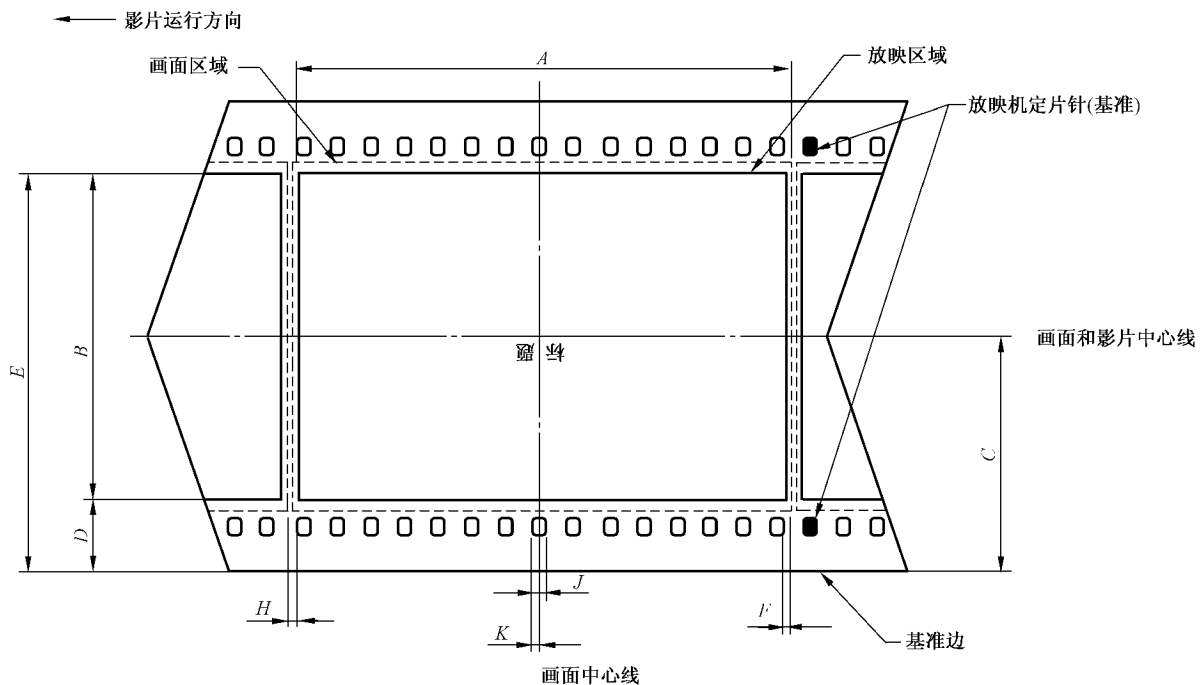
图 1 影片放映区域(朝向放映物镜,面对乳胶面一侧)
