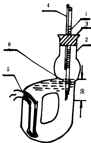
图1 电热熔点测定器
