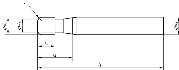
图1 型式1:短型圆弧立铣刀
