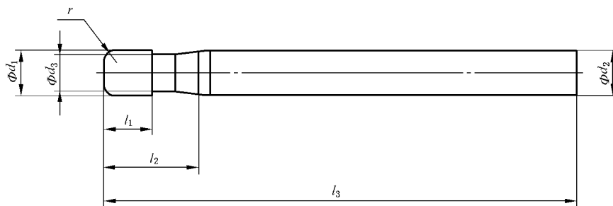
图2 型式2:长型圆弧立铣刀
