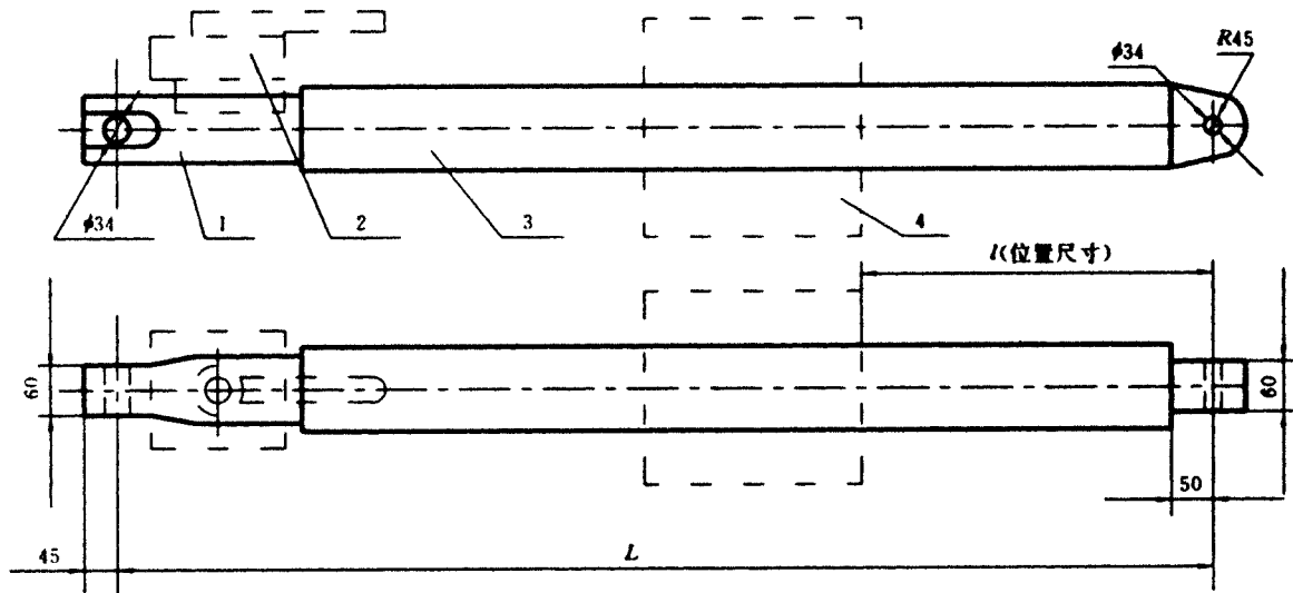
图 1 液压推溜器
