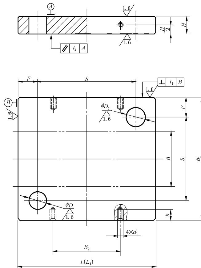
图 1 对角导柱下模座
