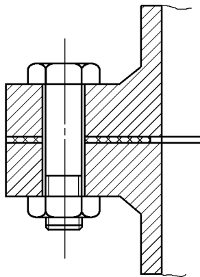
a) 全平面(FF型)法兰密封面及适用的垫片
