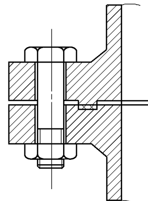
d) 榫槽面(TG型)法兰密封面及适用的垫片
