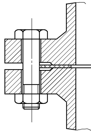
b) 突面(RF型)法兰密封面及适用的垫片
