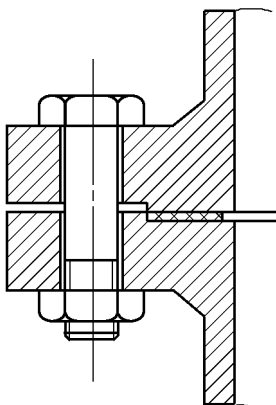
c) 凹凸面(MF型)法兰密封面及适用的垫片
