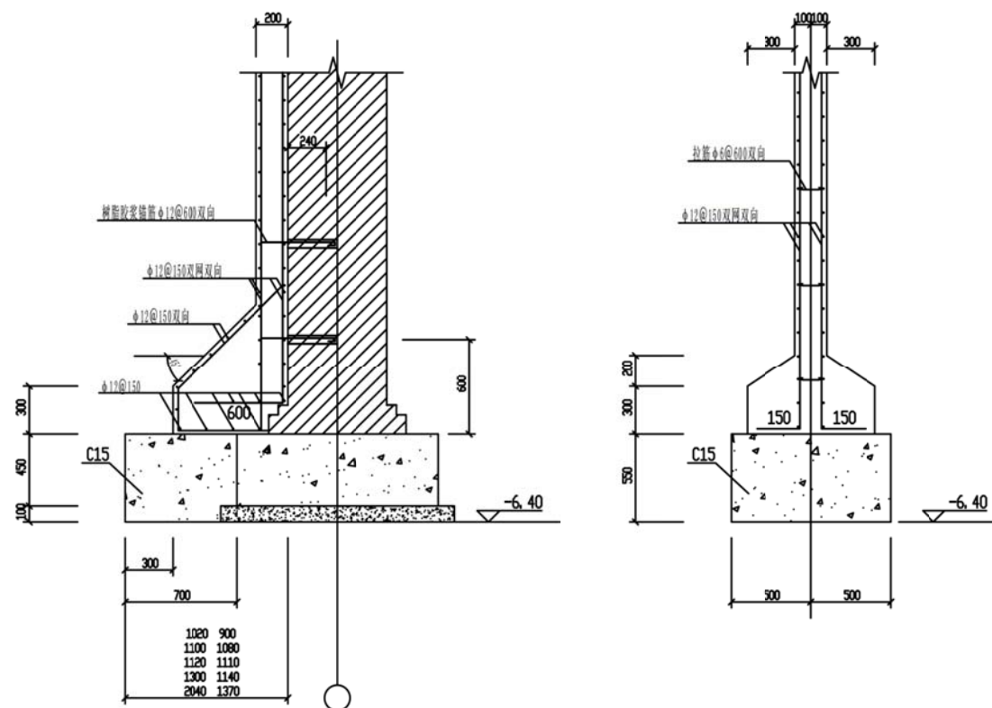
剪力墙基础配筋图
