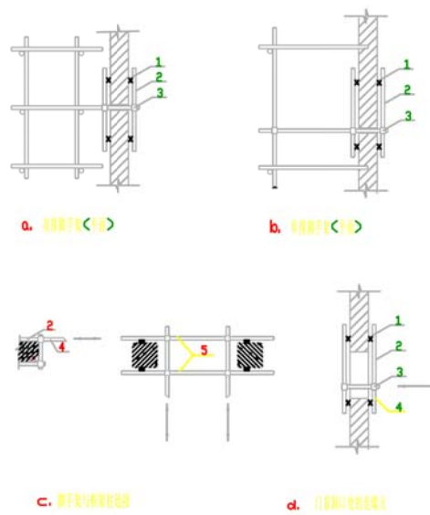
门框与墙体连接示意图
