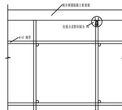
外架与框梁梁的拉接方案2
