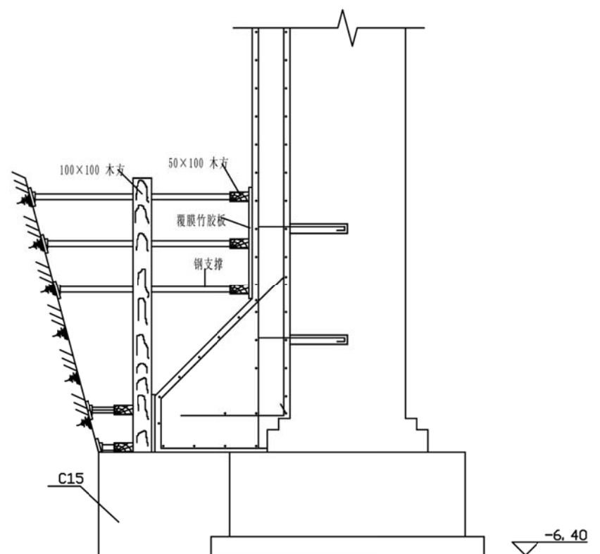
加固基础模板支设图
