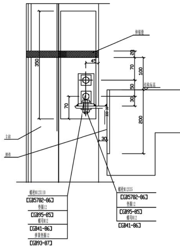
立柱安装节点
