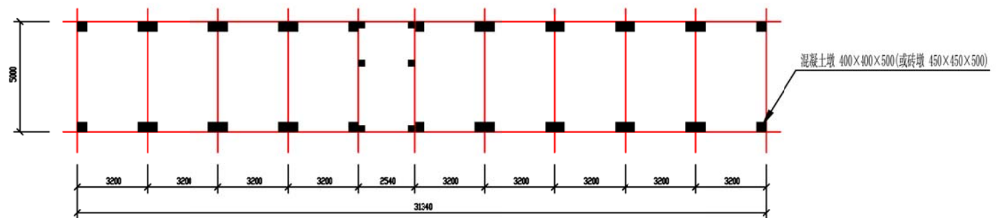
集装箱盒子办公室基础平面图
