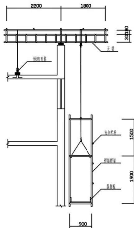
剪力墙结构外装修吊篮装配图
