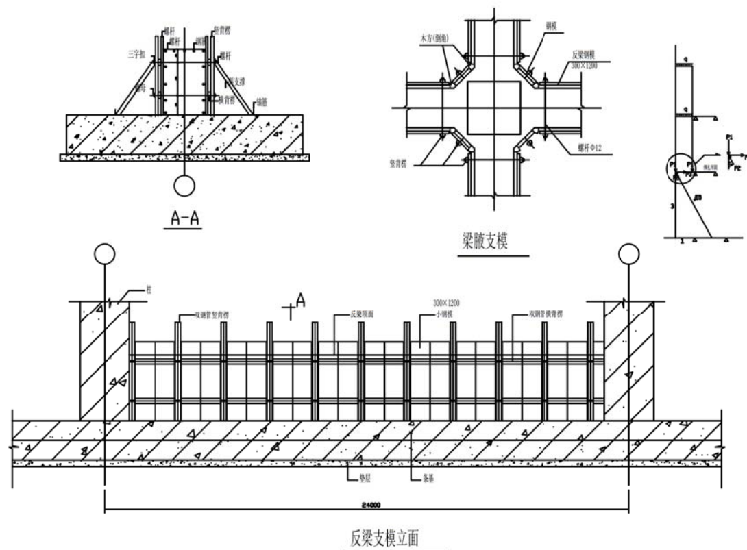
基础反梁支模图1
