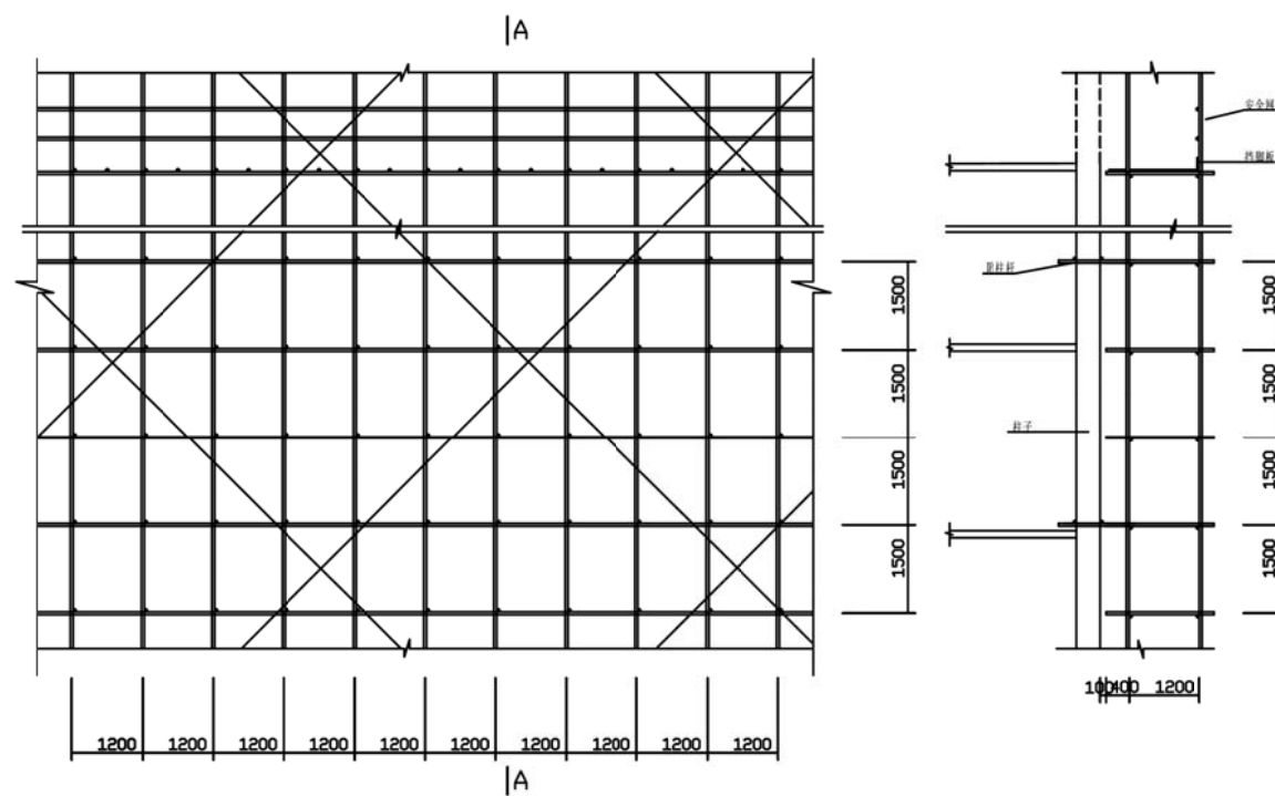
框架双排架脚手架图
