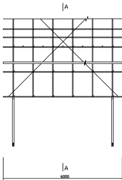
结构施工挂架立面图
