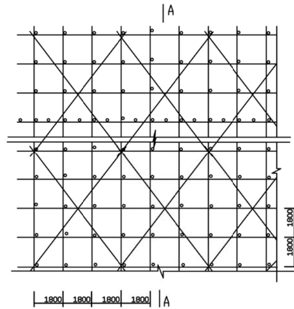
脚手架与结构拉结图
