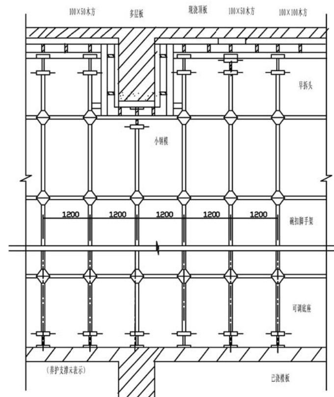
梁板碗扣式脚手架图
