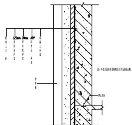
护坡桩支护外墙防水示意图
