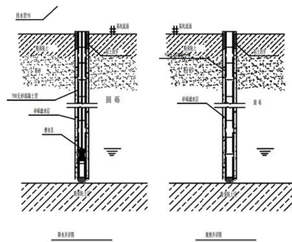
降水井及观察井详图
