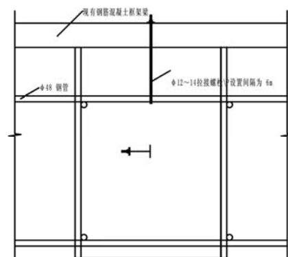
外架与框梁梁的拉接方案1
