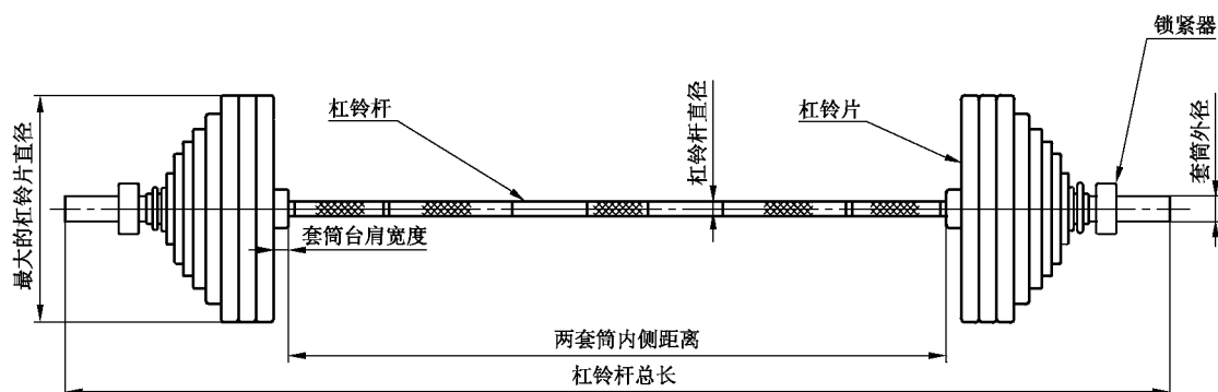
图 1 举重杠铃部件名称
