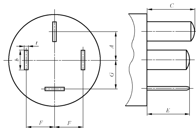
图 1 三相插头
