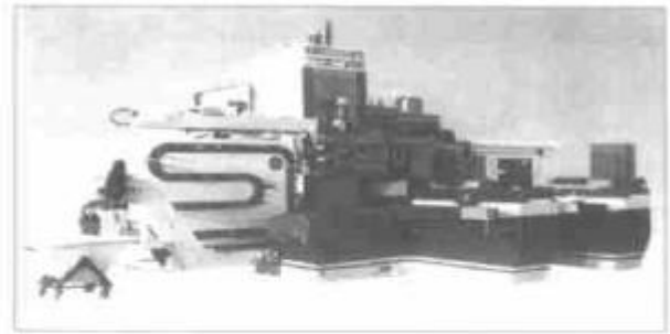
图 3 UD80 型换刀换箱柔性加工单元 Fig. 3 UD80 type flexible machining cell for tool changing and box changing
