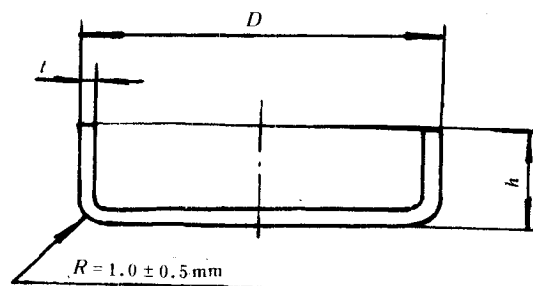
图 1 井型样品盘
