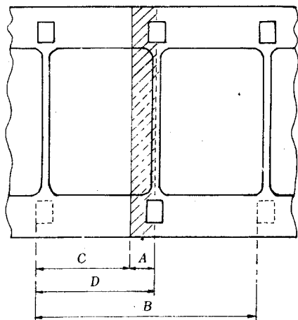
图 1 16 mm 影片洗印型接头
