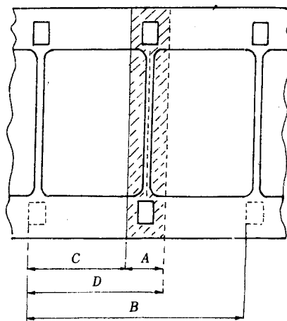
图 2 16 mm 影片放映型接头
