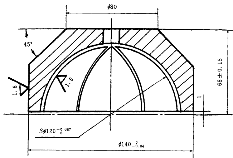
图 1 上球形衬套
