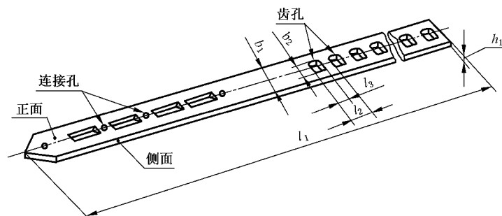
图1 剑杆带
