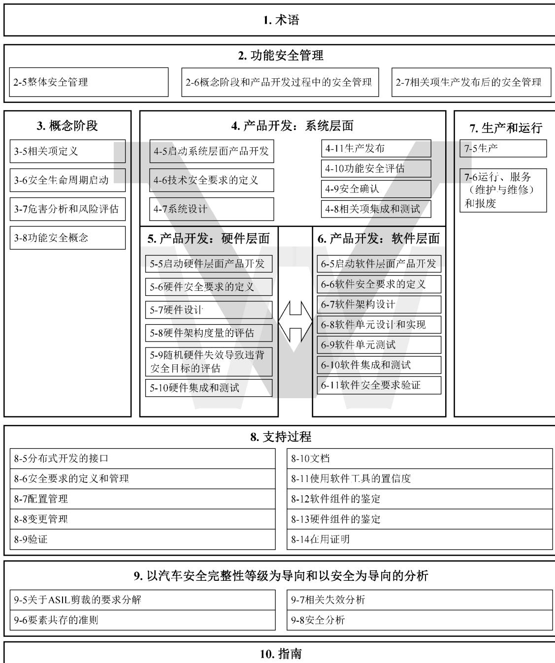
图 1 GB/T 34590—2017 概览
