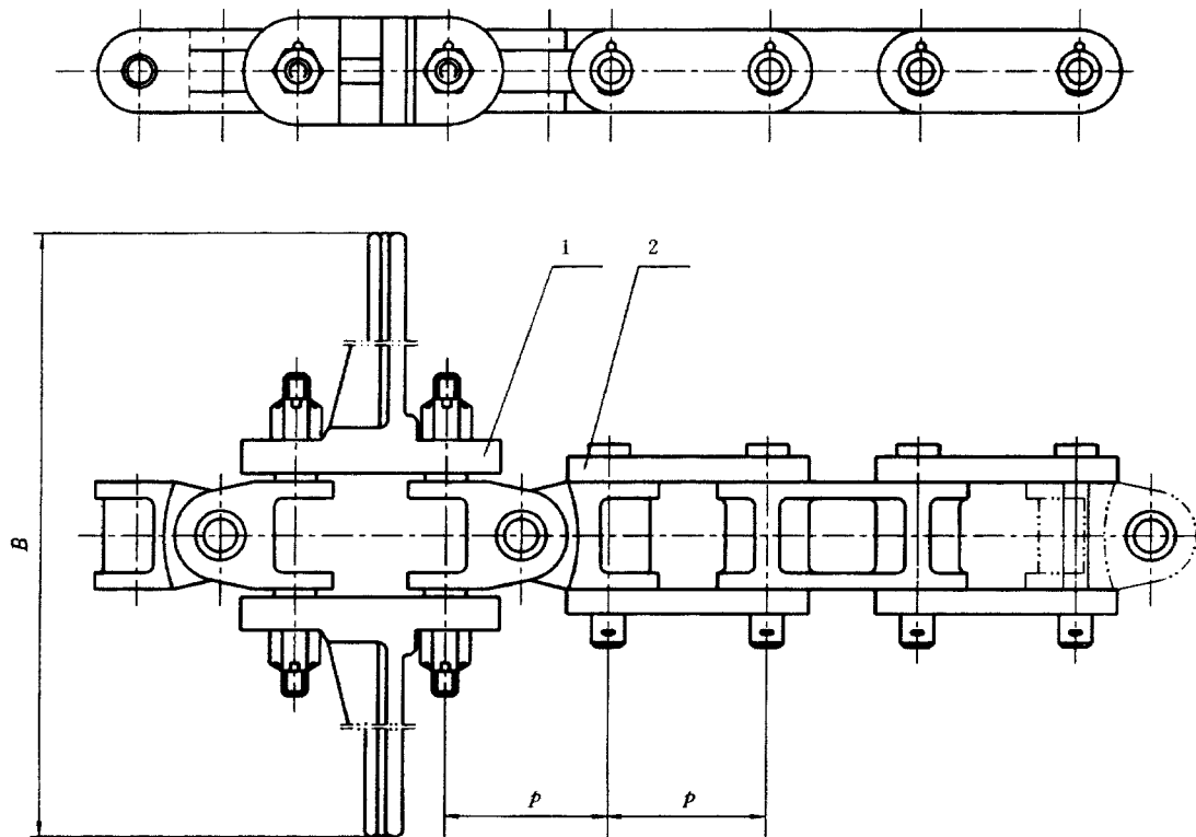
图1 整体链环式套筒刮板链 1—刮板节;2—链节
