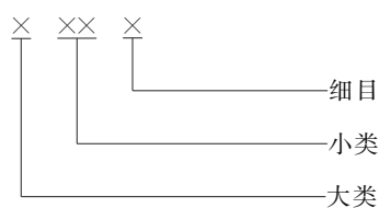
图 1 代码结构图
