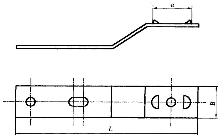
图 1 单向固定片结构示意图
