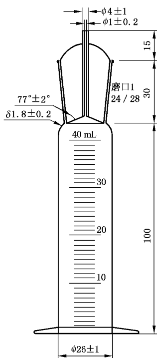
图 1 离子交换树脂密度计
