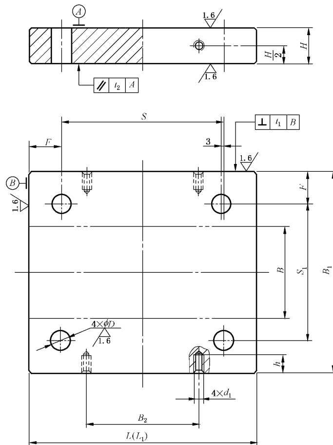
图 1 四导柱下模座
