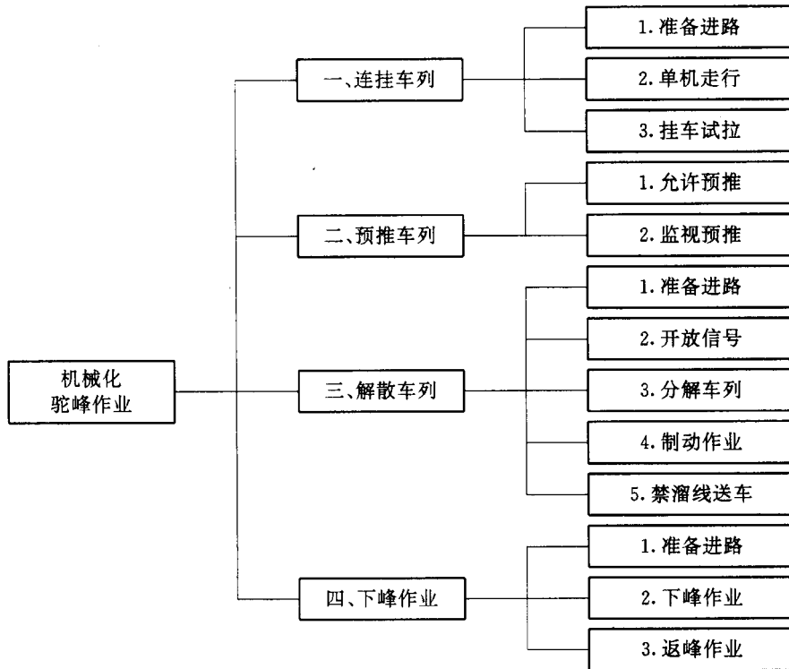
图1 铁路调车机械(半自动)化驼峰作业程序图
