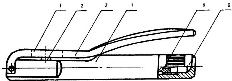
1—弹壳孔；2—底火座；3—手柄；4—压杆； 5—顶针；6—螺帽
