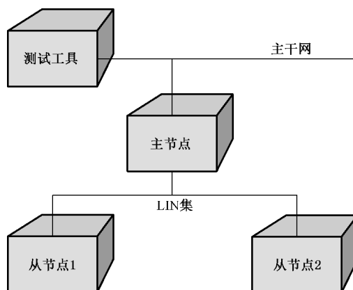
图 1 使用传输层的 LIN 集的典型系统设置
