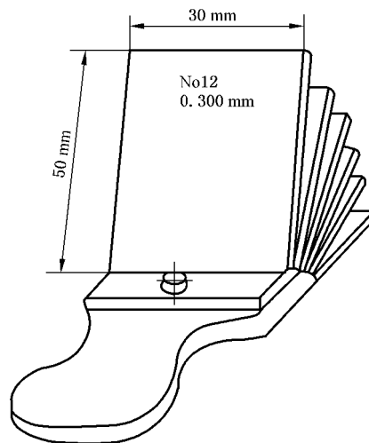
图2 B型隔距片 a
