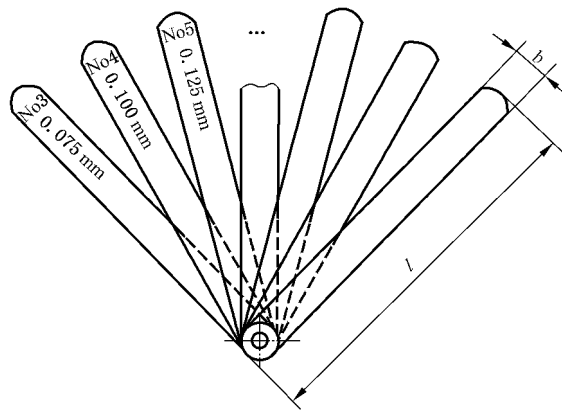
图1 A型隔距片 a
