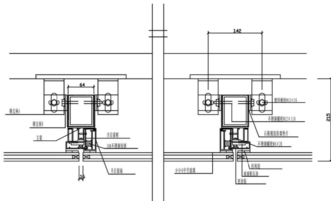
幕墙水平开启节点示意图
