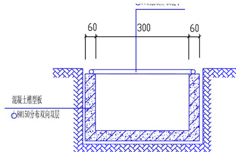
预制排水沟构造图
