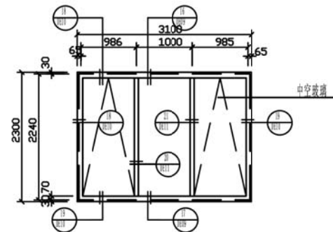
LC3123 合金窗
