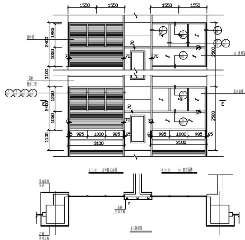
幕墙节点图5
