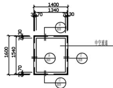
幕墙节点图6
