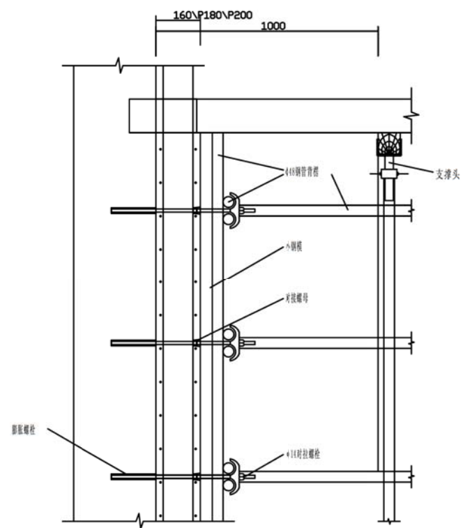
墙模板支设示意图方案2
