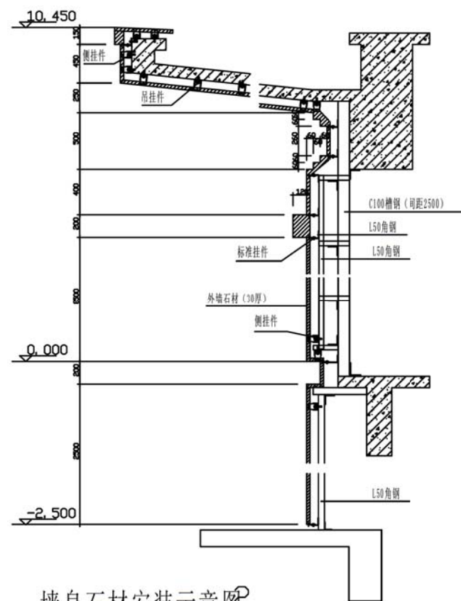
墙身石材安装示意图
