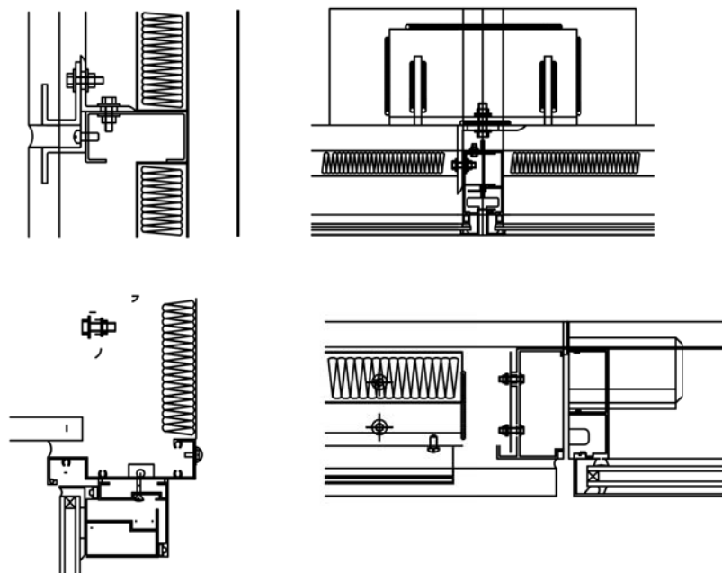
幕墙节点示意图
