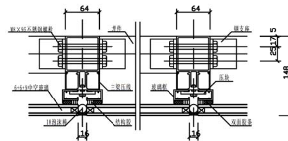
带形窗水平固定节点
