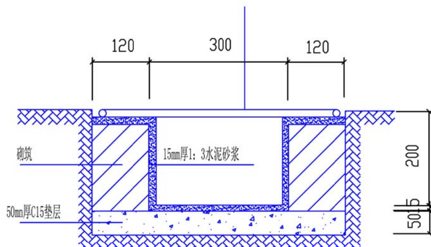
砌筑排水沟构造图
