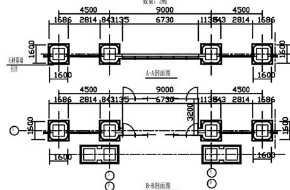
幕墙节点图4
