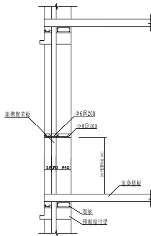
圈梁及过梁施工示意图
