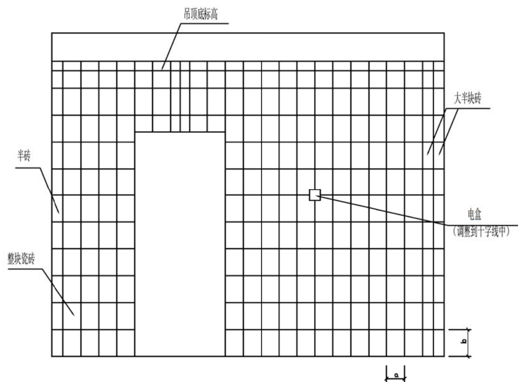
墙面排砖图2
