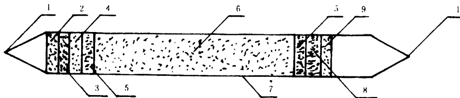
图 1 氧气检测管示意图
