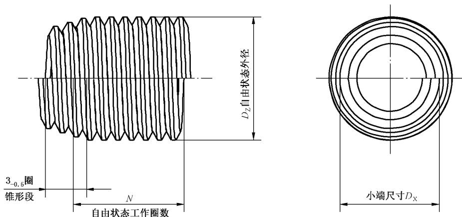
图 1 型式尺寸
