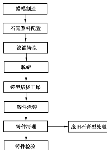
图 1 铝合金石膏型铸造工艺流程
