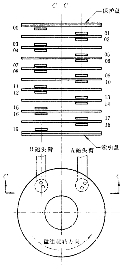
图1 记录面与磁头配置的示意图
