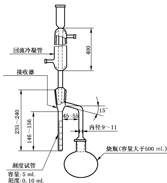
图 1 水分测定器
