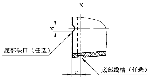
图 1 圆锥形筒管
