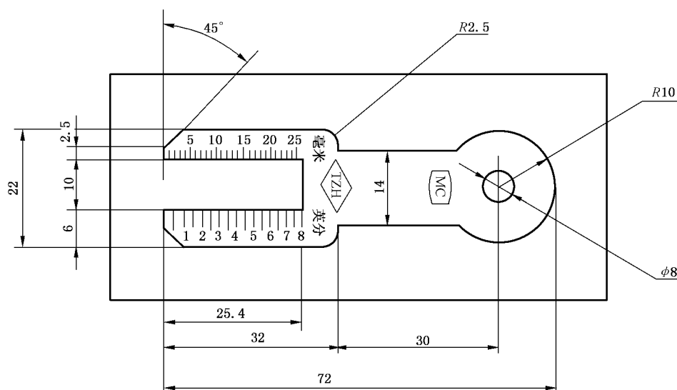
图 1 绒头长度量卡
