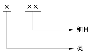
图 1 代码结构图
