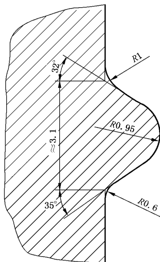
图 1 铣刀轮廓
