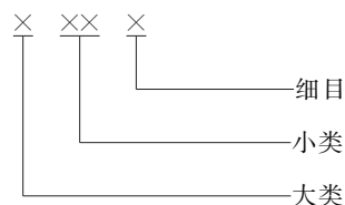
图 1 代码结构图
