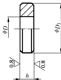
图 1 推板垫圈
