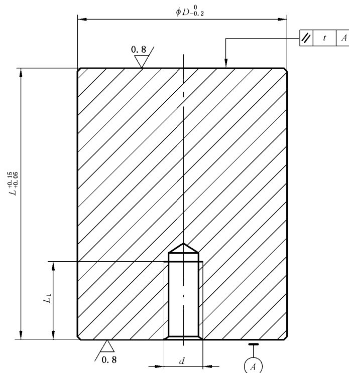
图 1 A 型支承柱
