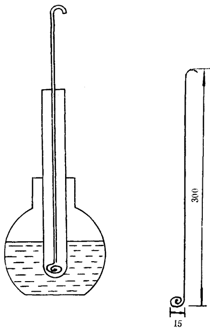
树脂固化时间测定装置图
