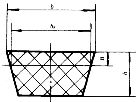
图 1 带的截面
