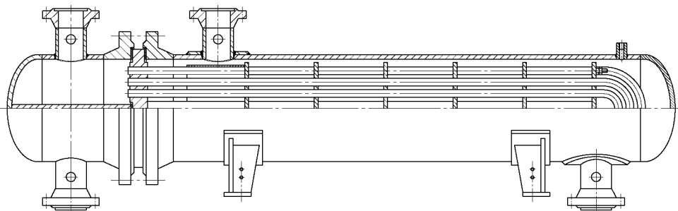
图 1 热交换器
