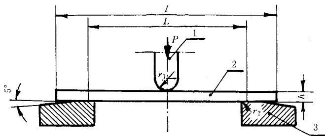
图 1 装置示意图
